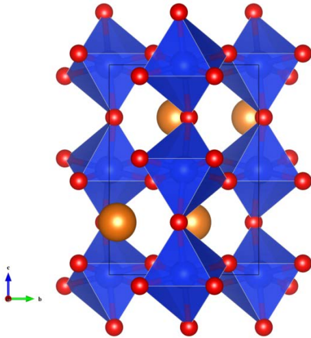
図1. ブリッジマナイトの結晶構造
