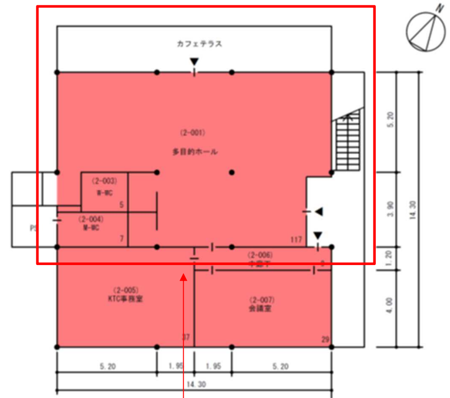
工学研究科ラーニングcommons平面図
