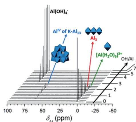
図3 定量 ^{27}\text{Al} NMRスペクトル 多様な溶液内化学種の多成分同時非破壊定量が可能である。
