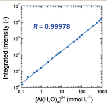
図2 定量 ^{27}\text{Al} NMR法の検量線 極めて広範囲の濃度領域で直線性が成立している。
