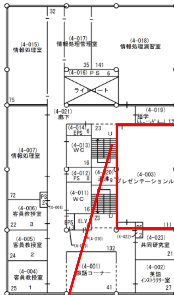
第五学舎4階平面図
