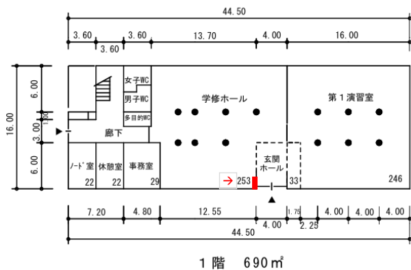
情報基盤センター（分館）1階 平面図
