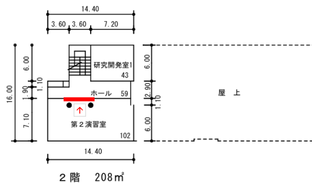
情報基盤センター（分館）2階 平面図
