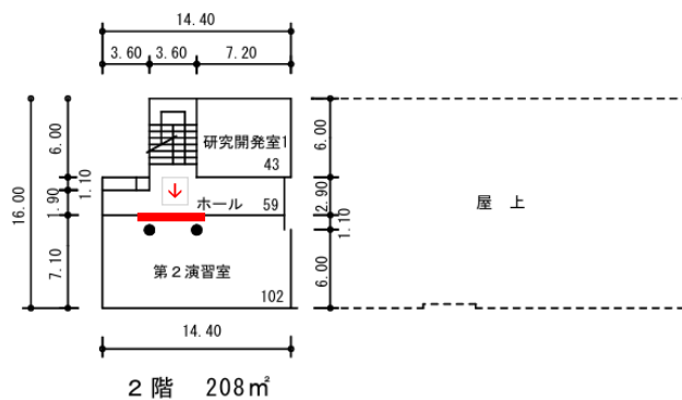
情報基盤センター（分館）2階 平面図
