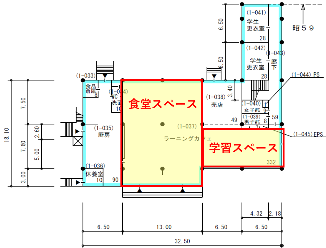
A棟 1階 平面図
