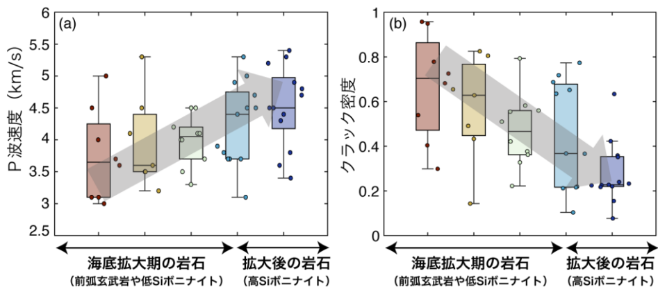
図 4 (a) 岩石種ごとの P 波速度の比較。図の左から右にかけて前弧地殻形成の初期から後期に形成された岩石の結果を示す。海底拡大後に形成された岩石は P 波速度が大きい。(b) P 波速度と空隙率などから推定された岩石種ごとのクラック密度。P 波速度のバリエーションは、岩石に含まれるクラックの量の違いで説明できることがわかった。
