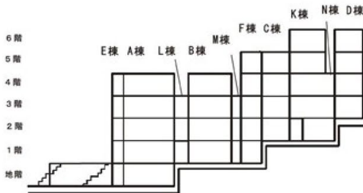
南 北 学生用掲示板 横断面
