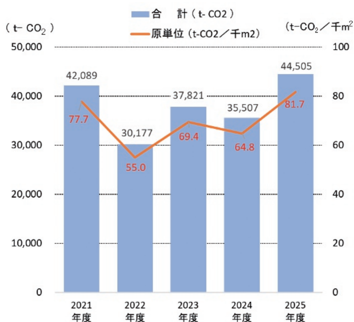
図2 CO 2 排出量
